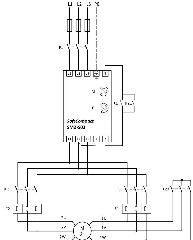
SoftCompact® SM2-S03 Anschlussempfehlung für Sanftanlauf mit polumschaltbaren Motoren (z.B. Dahlander) Recommended connection for soft-start with pole-change motors (e.g. Dahlander)
