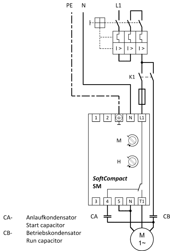
SoftCompact® SM Anschlussempfehlung für Sanftanlauf Recommended connection for soft starting
